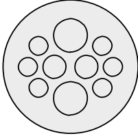
KEL-DP 32|10 A gy okrągły
